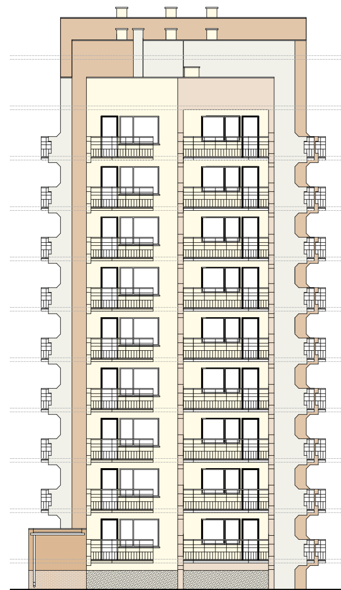
ELEWACJA POŁUDNIOWA
